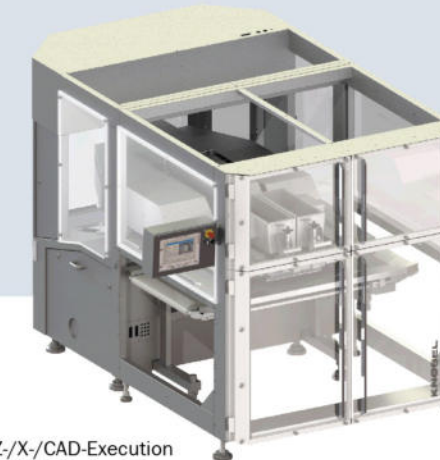
Z-/X-/CAD-Execution Z-/X-/CAD-Ausführung
