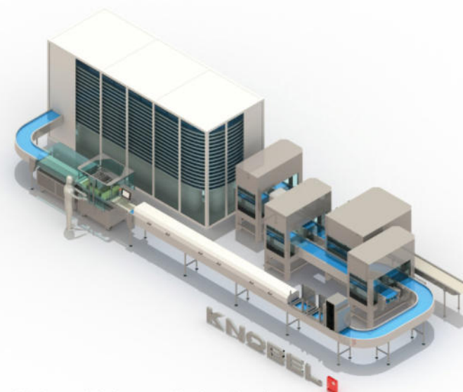
Step 3: Ergänzung mit Ausformung und Leerformenkontrolle mit automatischem Formenwechsler
